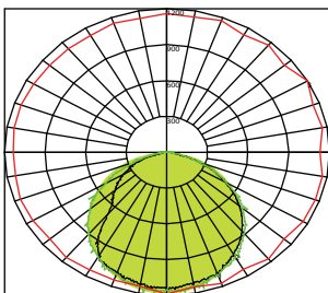
CURVA FOTOMÉTRICA
