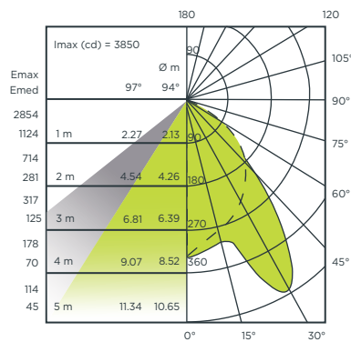
CURVA FOTOMÉTRICA 3 X 28W
