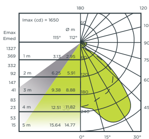
CURVA FOTOMÉTRICA
