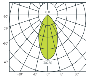
CURVA FOTOMÉTRICA
