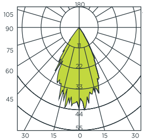
CURVA FOTOMÉTRICA
