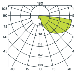
CURVA FOTOMÉTRICA
